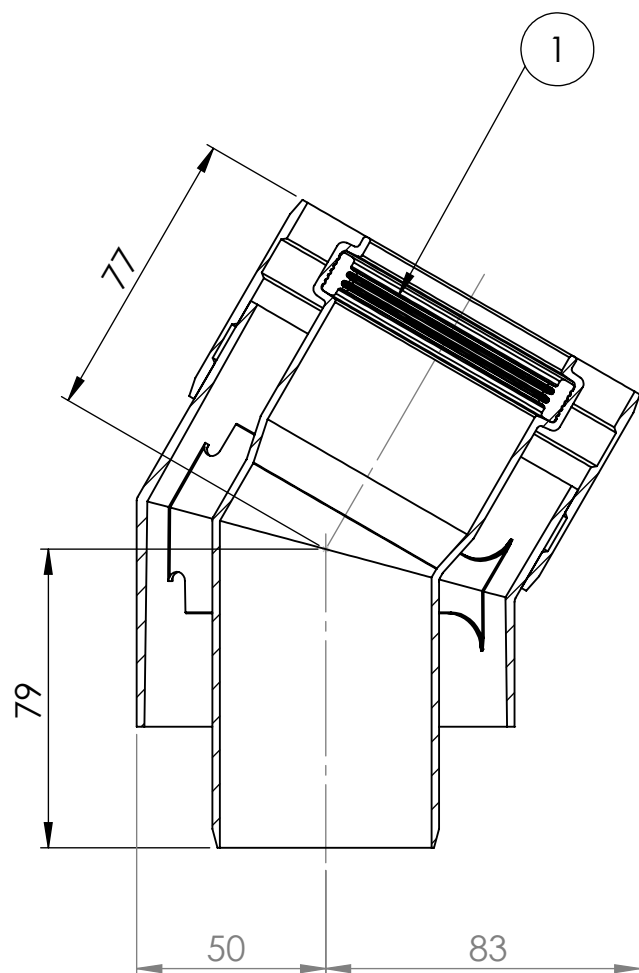
A-A (1 : 2)
